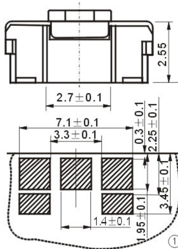
P.C.B LAYOUT
